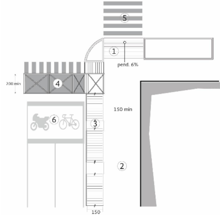
40 PLANTA DE PUENTE PEATONAL
