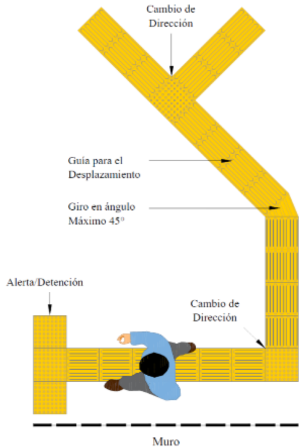
119 VARIANTE DE PANEL DE CAMBIO DE DIRECCIÓN (1 MÓDULO)
