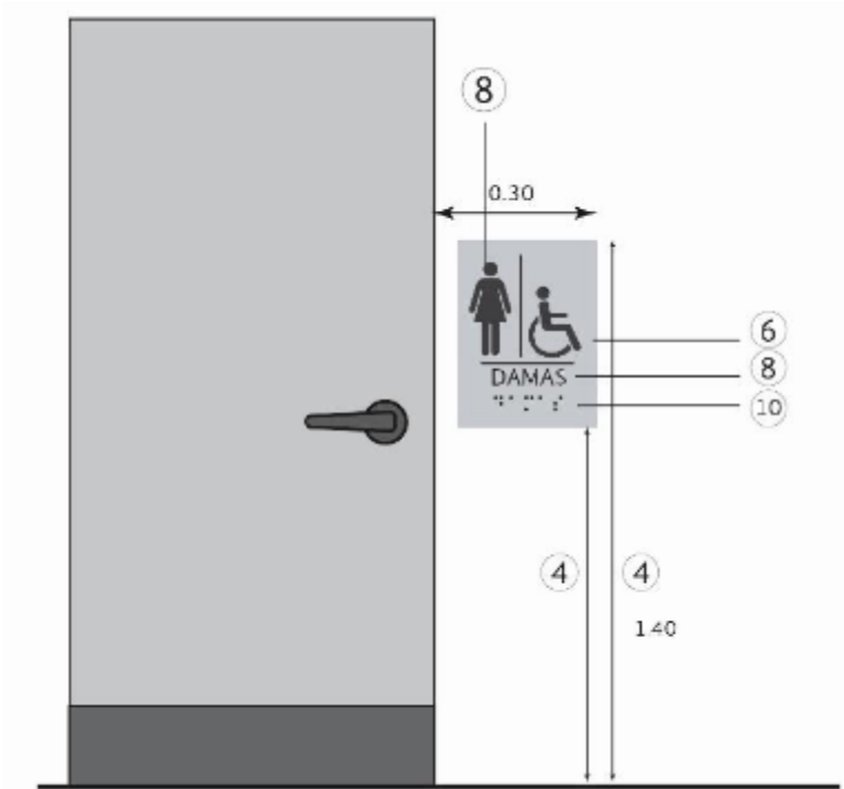
111 ESQUEMA PARA COLOCACIÓN DE PLACA
