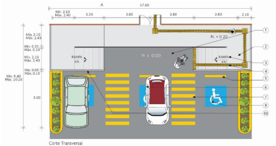
45 PLANTA PARA CAJÓN DE ESTACIONAMIENTO
